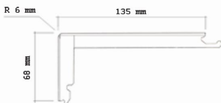
Profil hladký
