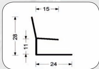
31263 Rohový profil 10 mm
