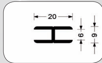
30224 H Spojovací profil
