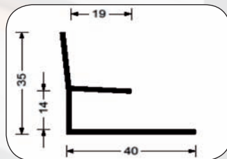
31007 Spojovací profil 13 mm
