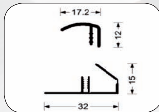
32192 Speciální profil Nr. 3
