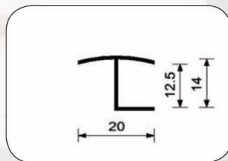
31228 Polo H - profil 13 mm
