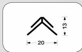
38282 Profil pro vnější roh
