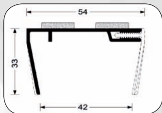
32309 Spojovací profil s lepidlem
