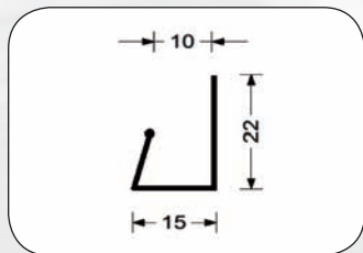
32306 U-Profil
