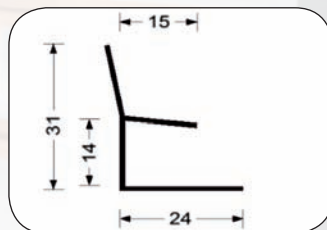
31209 Rohový profil 13 mm
