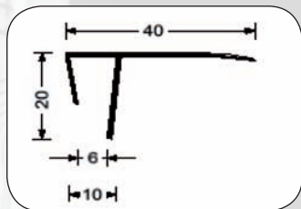
32378 F-Profil 40 mm
