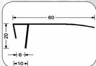
32351 F-Profil 60 mm
