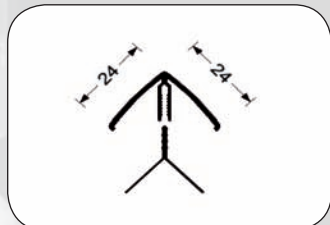
32190 Speciální profil Nr. 1
