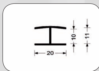
31259 H-Profil 10 mm
