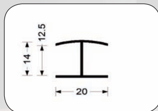
31208 H-Profil 14 mm
