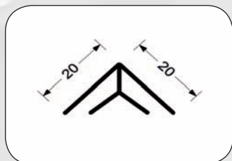
38313 Profil pro vnitřní roh
